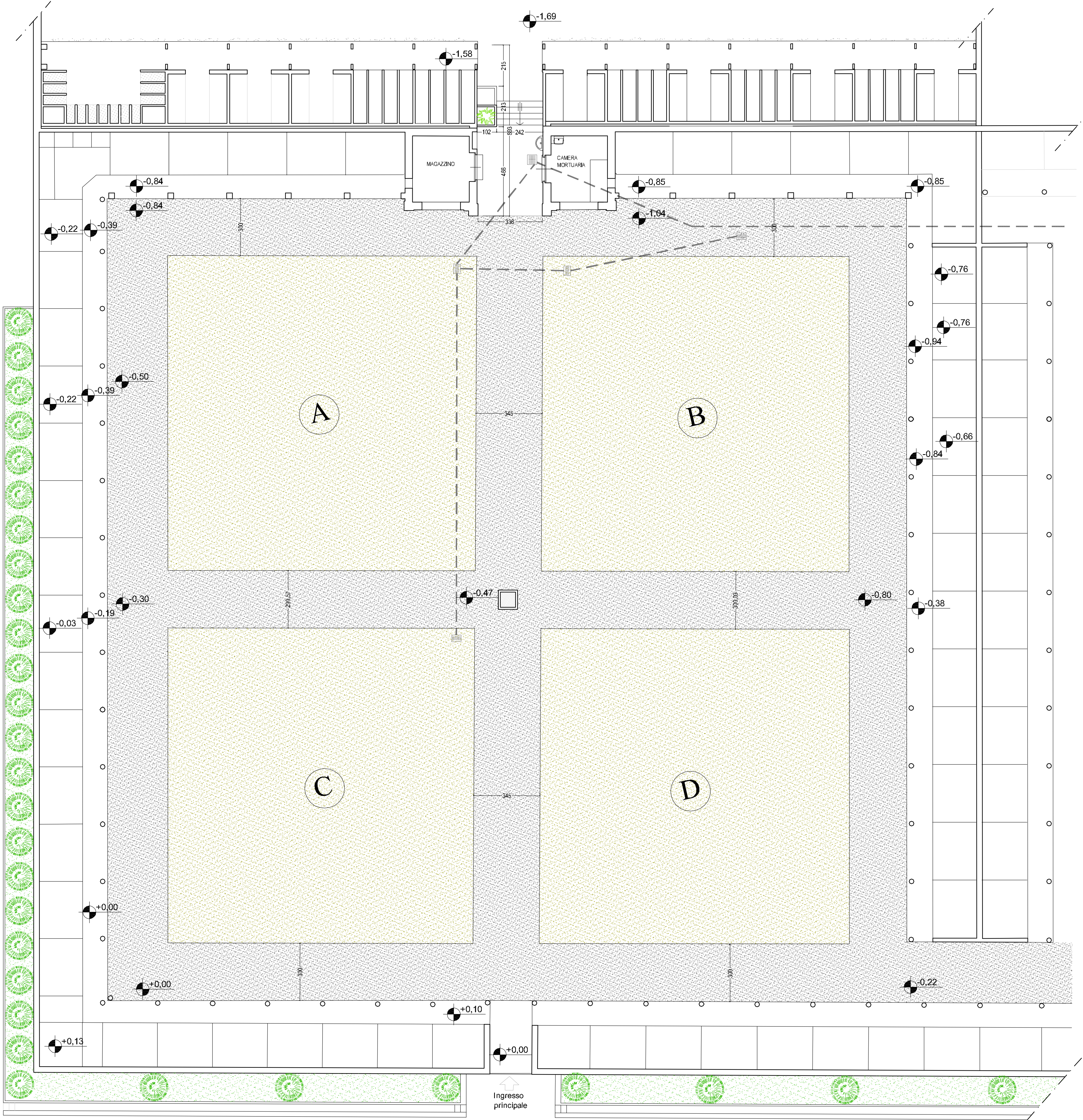
PLANIMETRIA - scala 1:100
