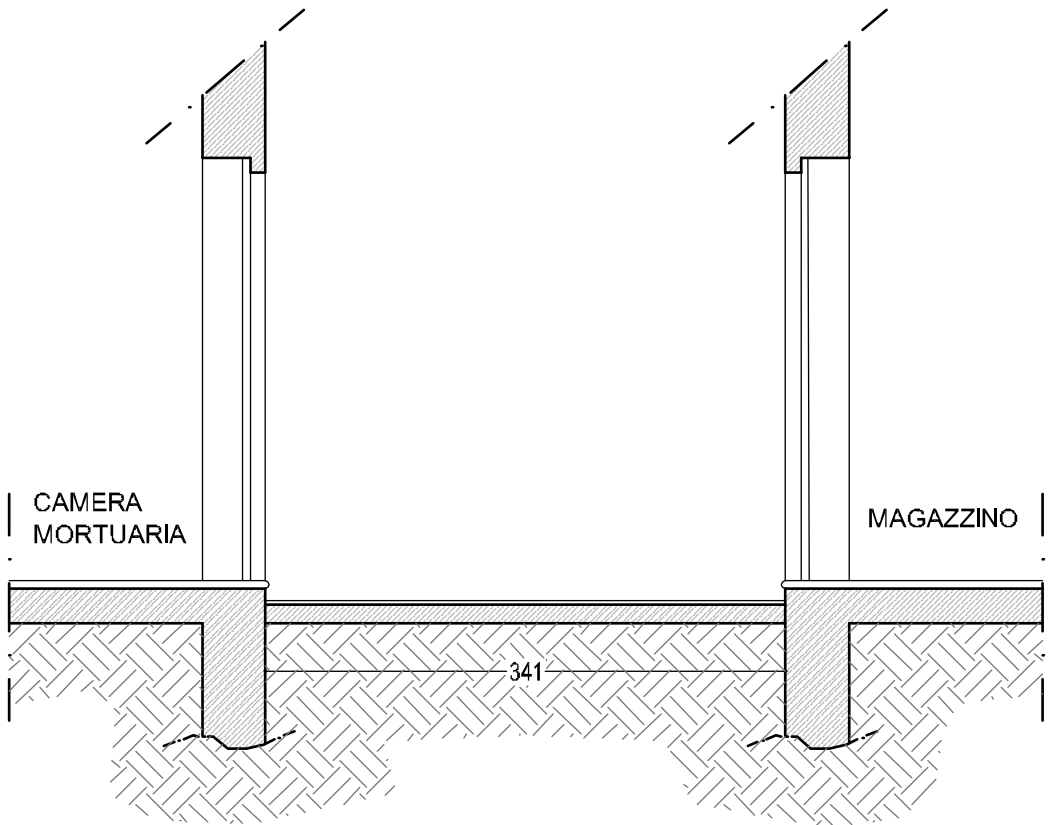
SEZIONE C-C
