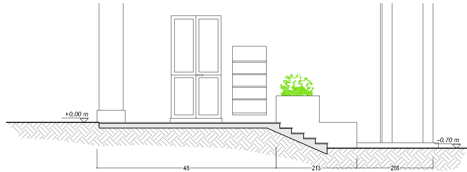
SEZIONE A-A
